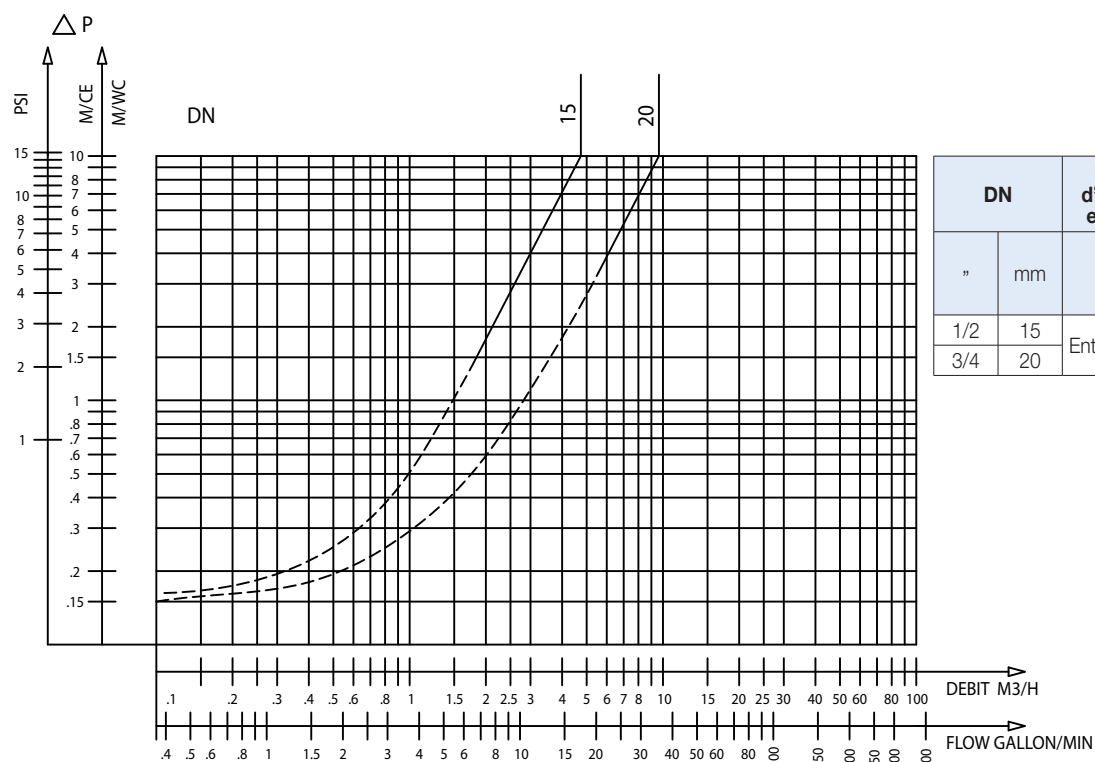
W - Abaque des pertes de charge
